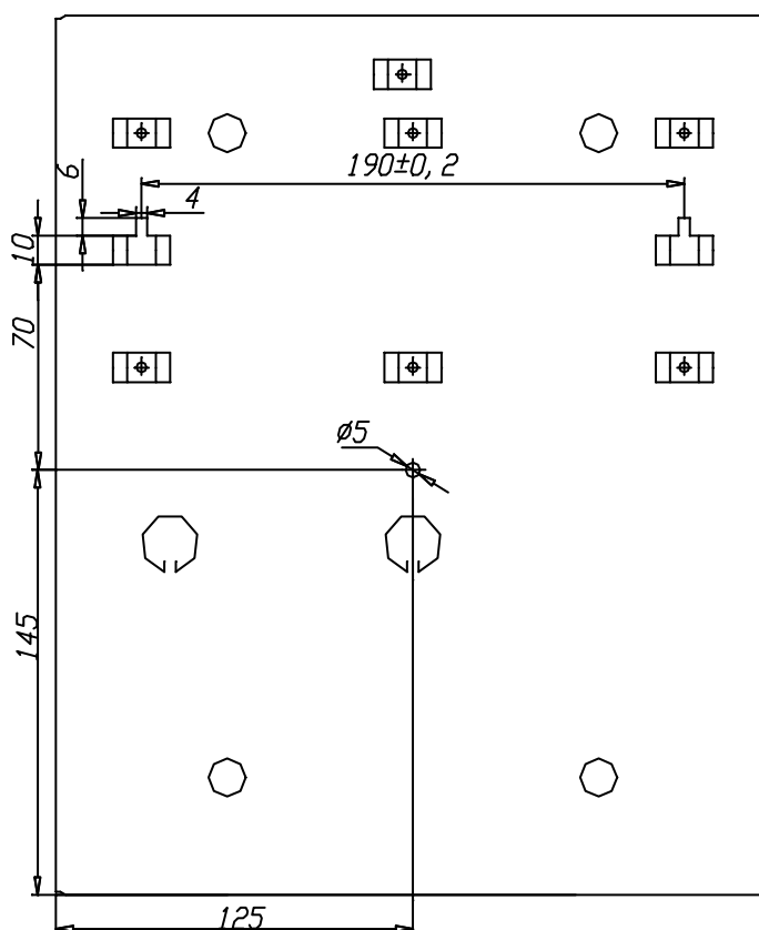
Установочные размеры
