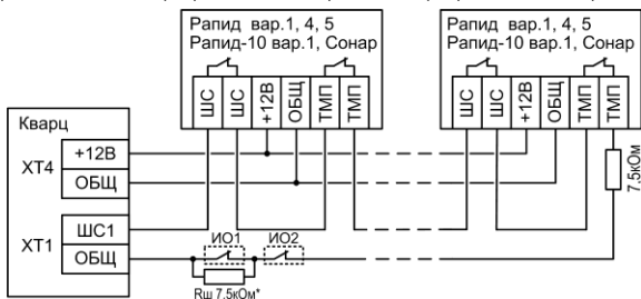
Рис.А9 Схема подключения охранных извещателей Рapid var.1,4,5, Рapid-10 var.1, Сонар, ПОЛЮС-2 (ИО1, ИО2)
