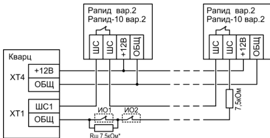
Рис.А8 Схема подключения охранных извещателей Рapid var.2, Рapid-10 var.2, ПОЛЮС-2 (ИО1, ИО2)
