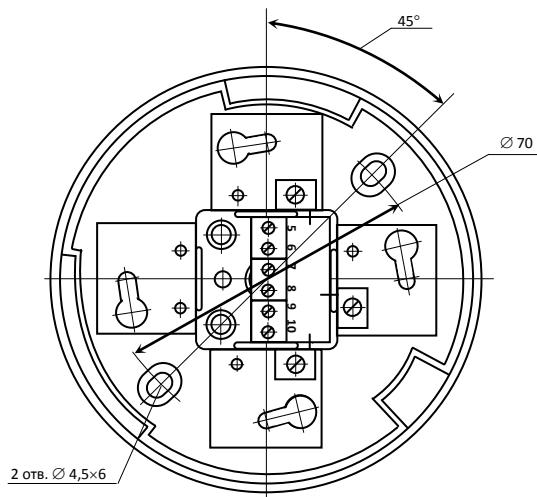
Рисунок 6 - Общий вид розетки с установленным модулем МС-01 (МС-02)
