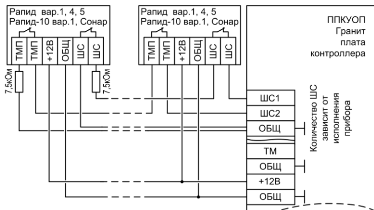
Рис.Б3 Схема подключения охранных извещателей Рapid вар.1,4,5, Рapid-10 вар.1, Сонар (тампер подключён к отдельному ШС)
