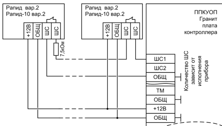
Рис.Б4 Схема подключения охранных извещателей Рapid вар.2, Рapid-10 вар.2
