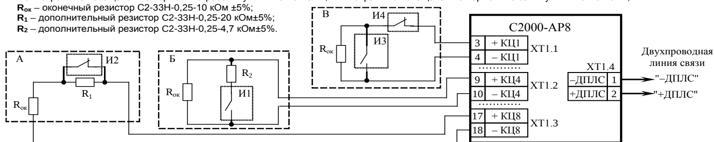
Рисунок 1 Схема соединений
